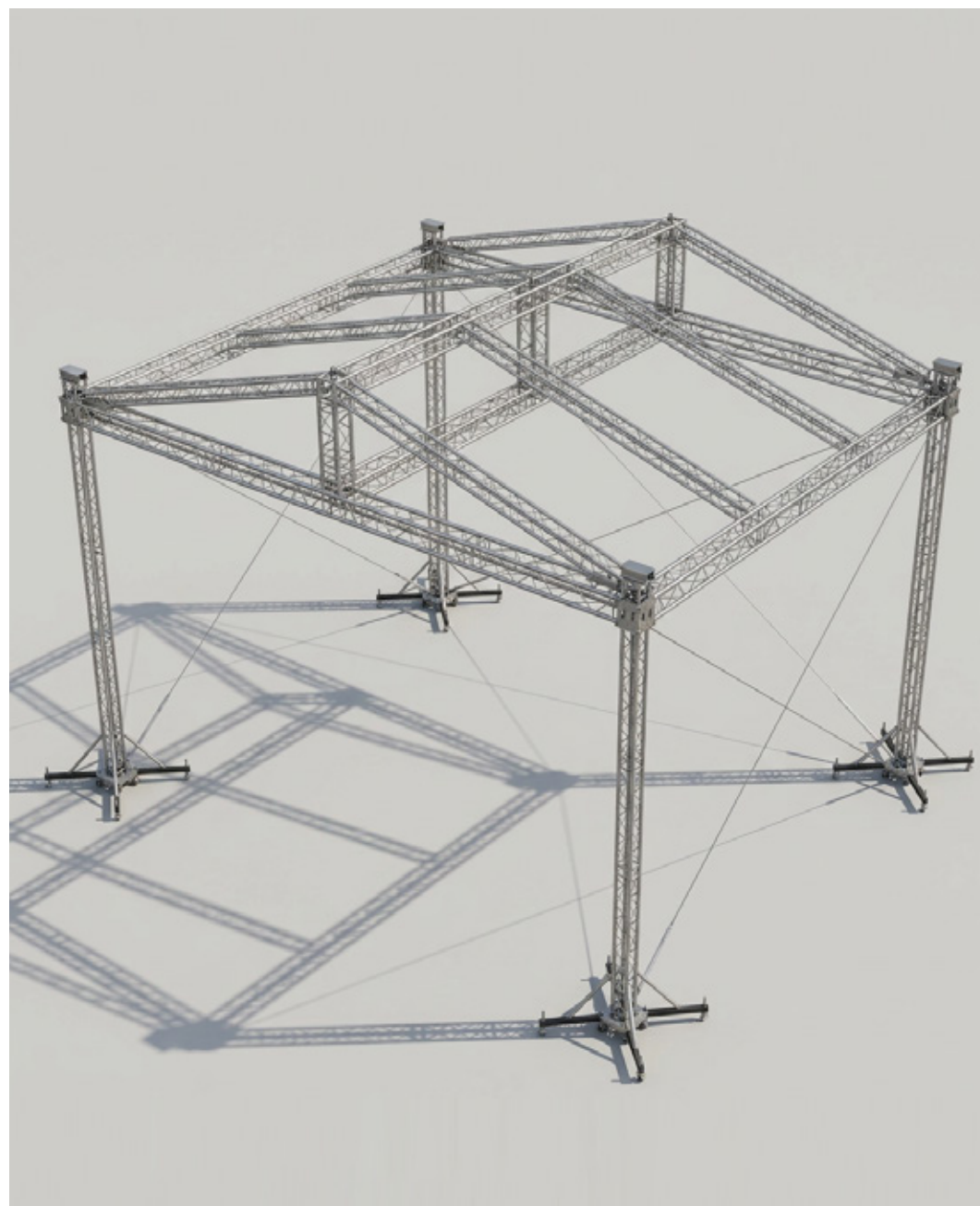
Techo 12*12 en truss
